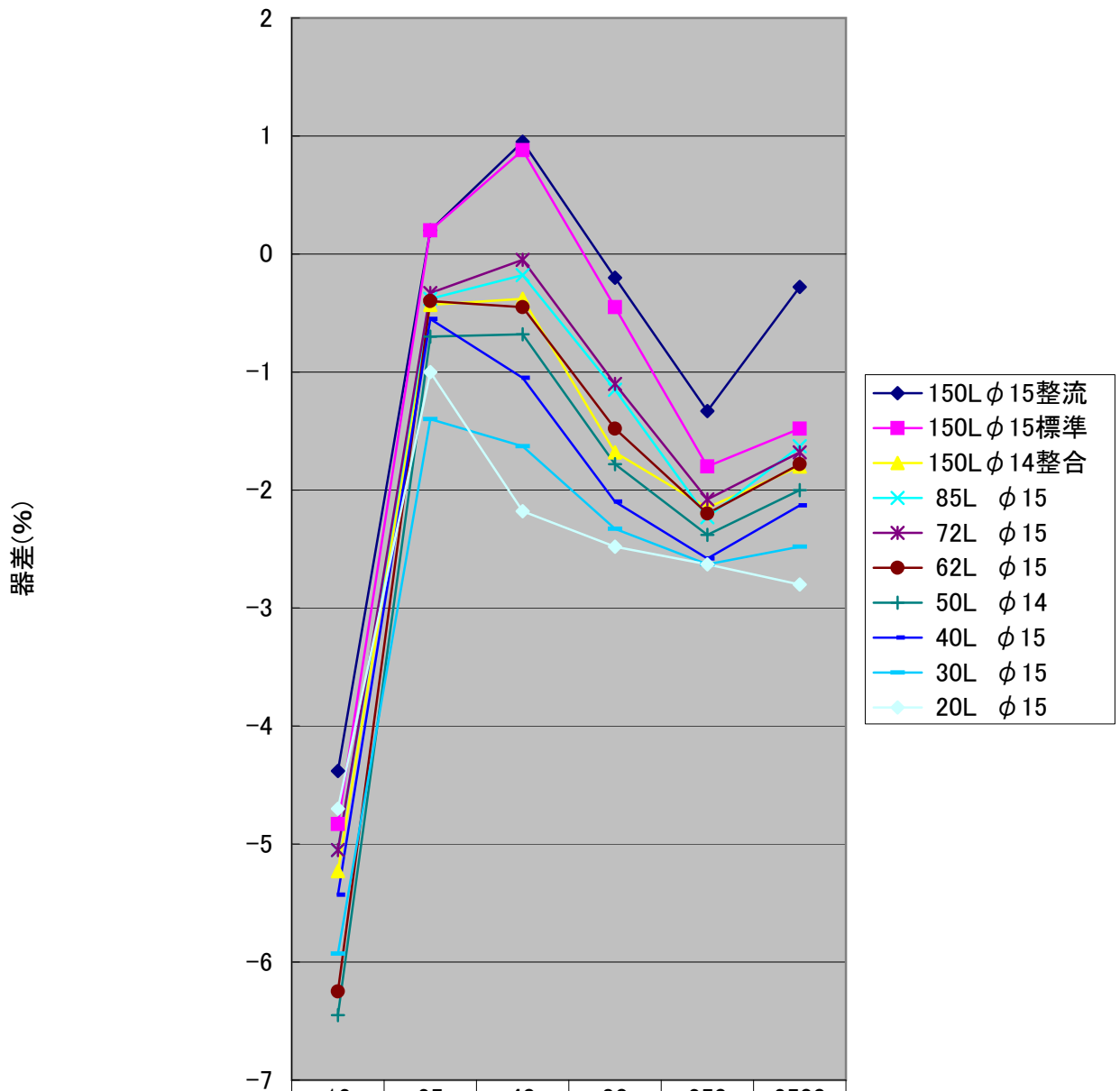
連結継手の種類と器差 13mmショート
